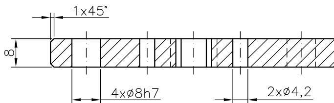
ŘEZ A-A
